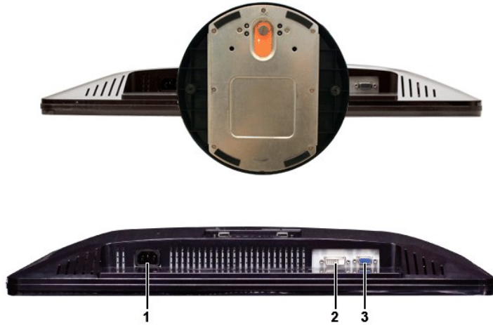
底視圖
