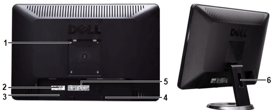
背視圖
